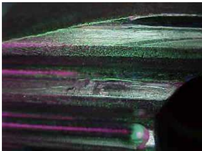
Found crack Magnaflux inspection. セッション磁気探傷検査、クラック発生。
